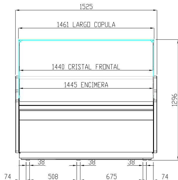
VISTA ALZADO
