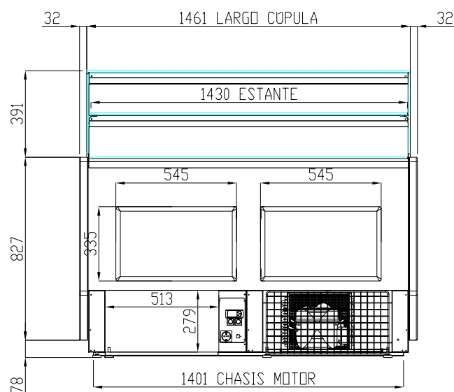
VISTAS TRASERA
