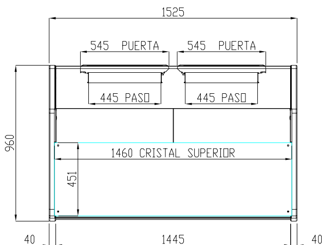
VISTA PLANTA
