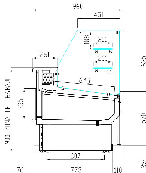
SECCIÓN DE PERFIL
