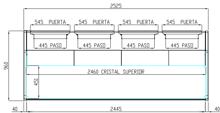
VISTA PLANTA
