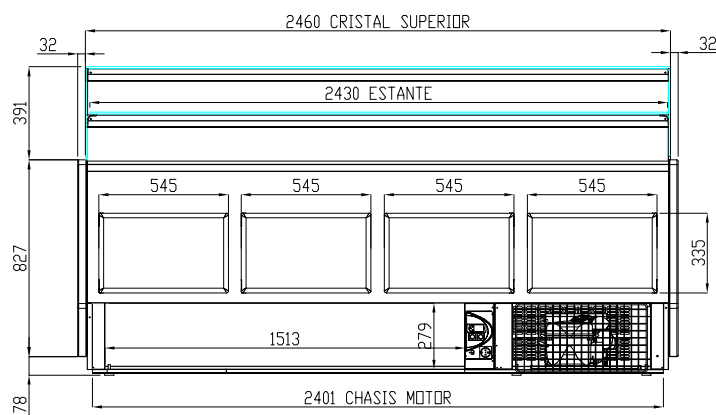
VISTAS TRASERA
