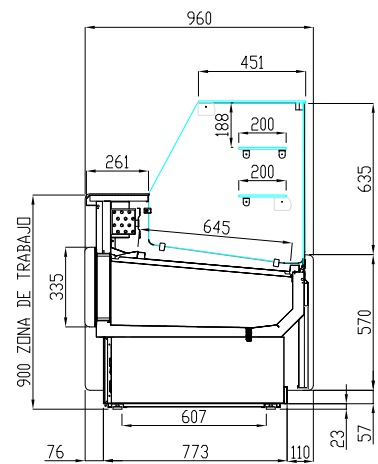
SECCIÓN DE PERFIL
