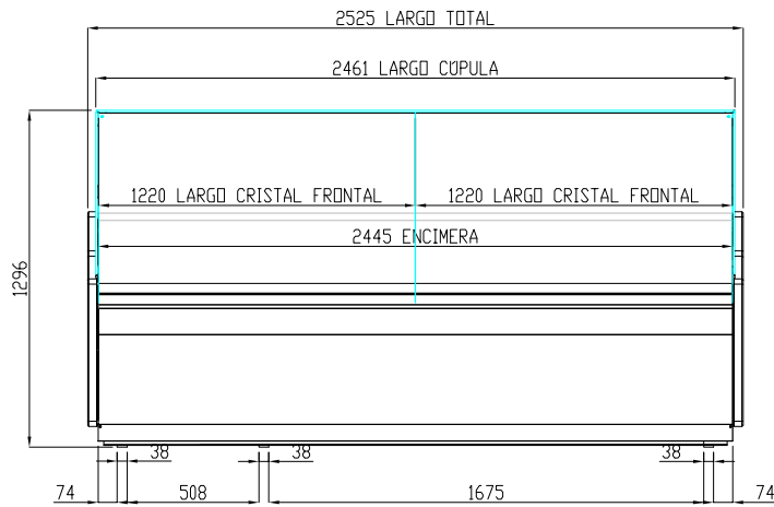
VISTA ALZADO
