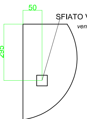
DETTAGLIO A Detail A
