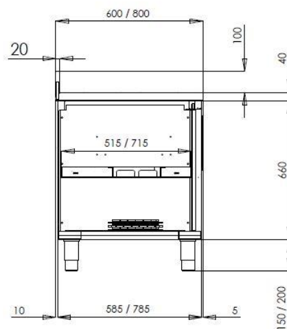
SEZIONE A-A
