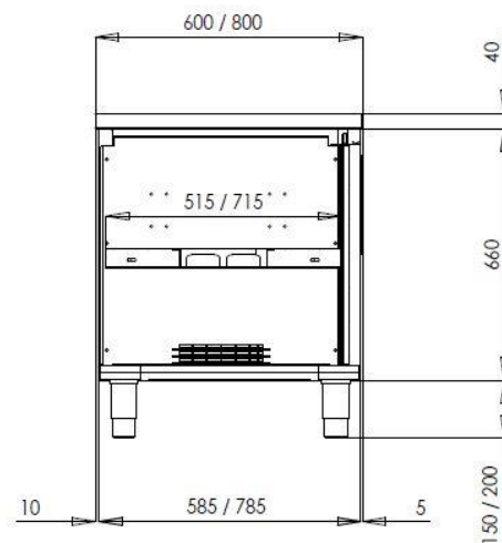
SEZIONE A-A
