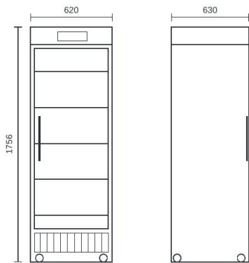
Front- und Seitenansicht · Gesamtmaße in mm
