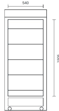
Frontansicht mit Innenmaßen
