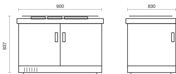
Vorder- und Seitenansicht · Gesamtmaße in mm
