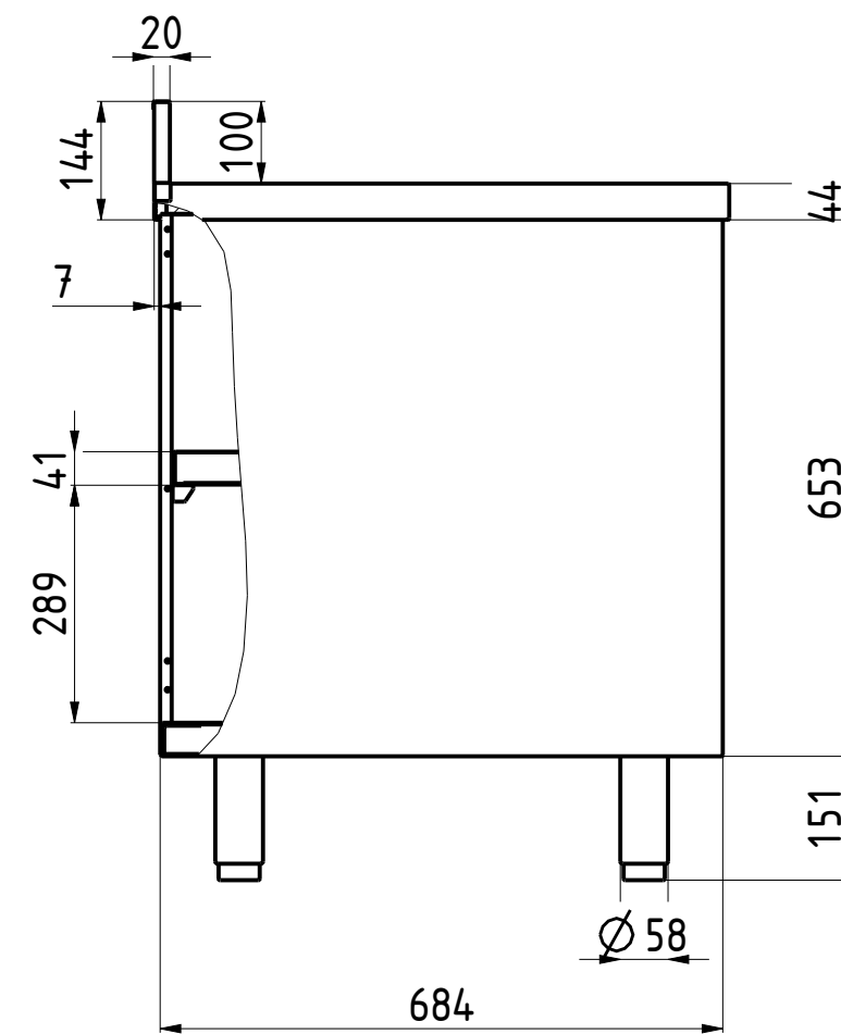
A-A
