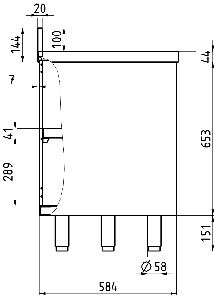
A-A
