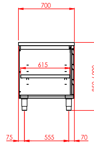
SEZIONE A-A
