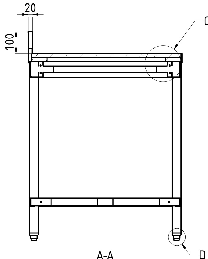
A-A
