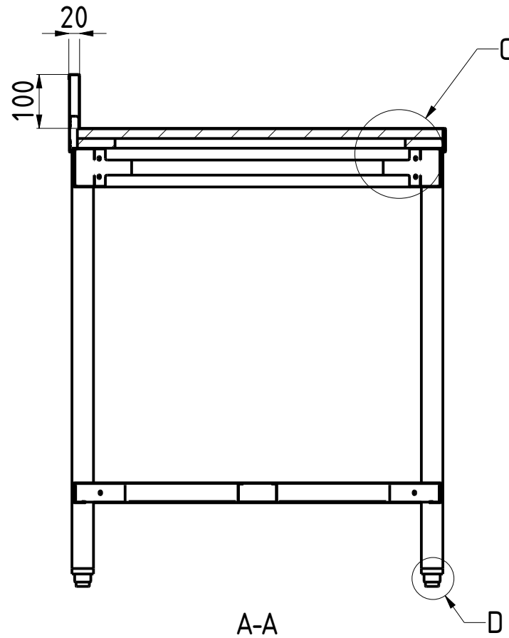
A-A
