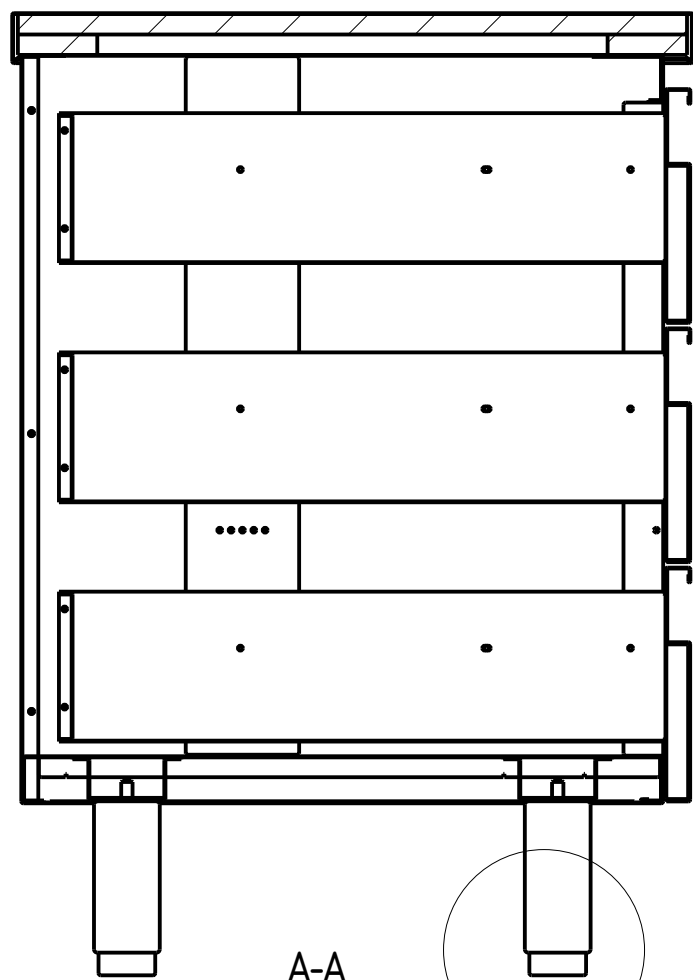
A-A
