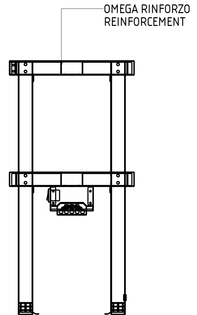
B-B
