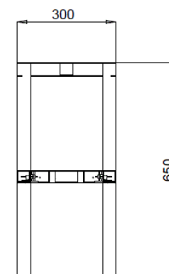
SEZIONE A-A
