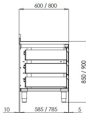
SEZIONE B-B
