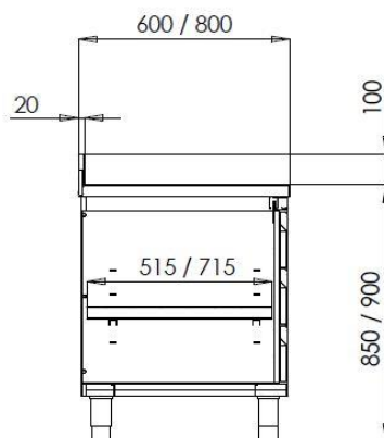
SEZIONE A-A
