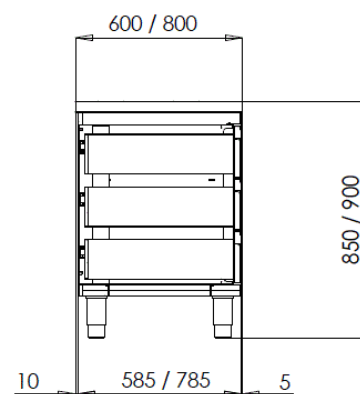
SEZIONE B-B
