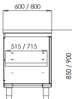
SEZIONE A-A
