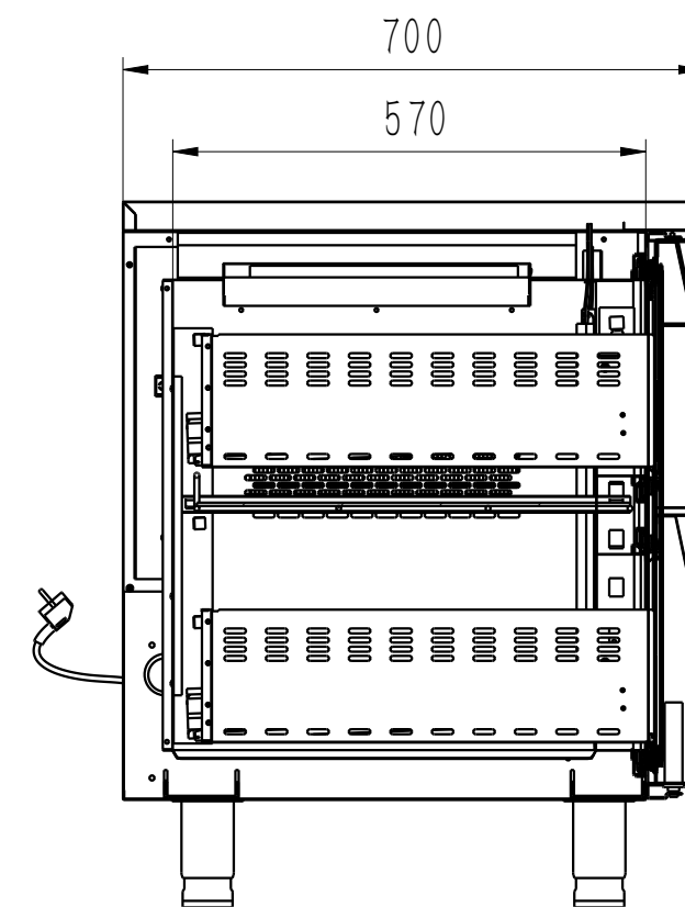
截面 A-A
