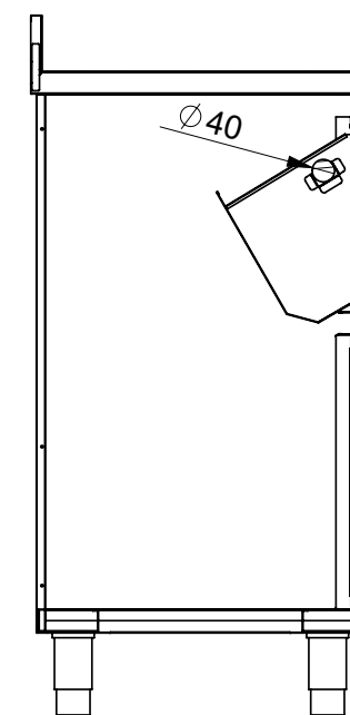
SEZIONE B-B
