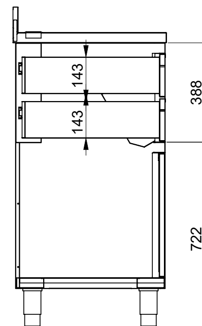
SEZIONE A-A
